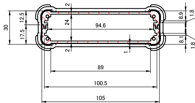
A-A (1:2)
